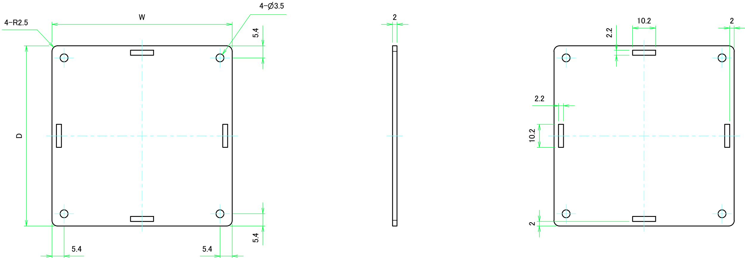
上カバー裏面 / Top cover Backside
