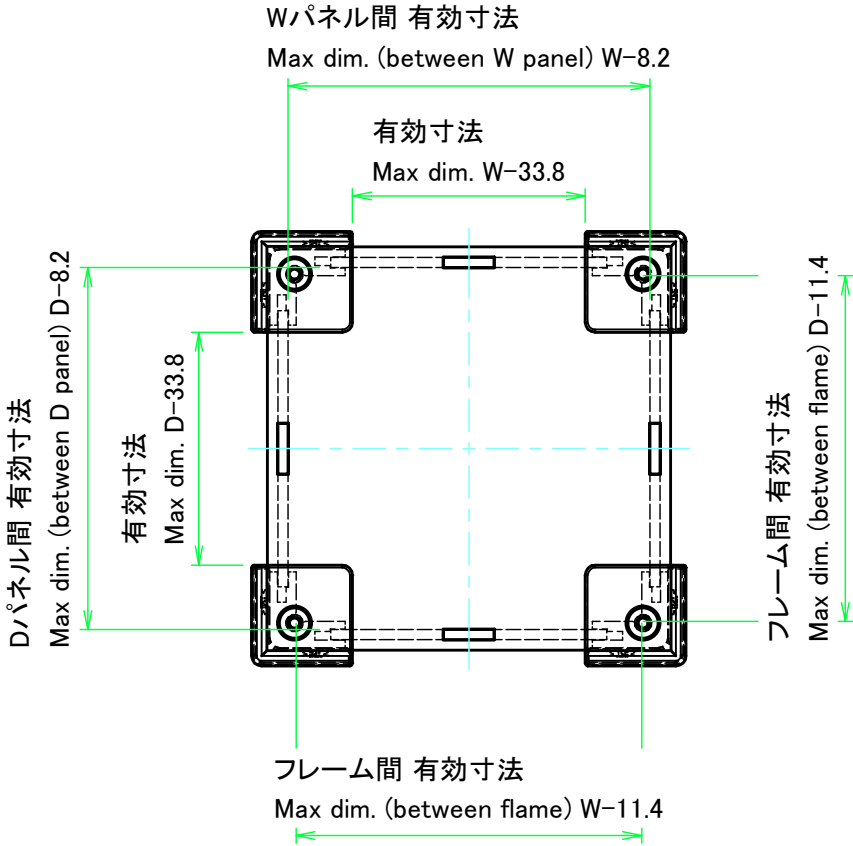
下カバー / Bottom cover
