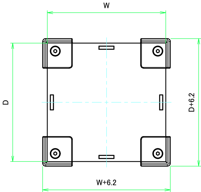
上カバー / Top cover
